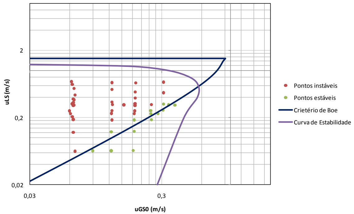
Figura 18 - Mapa de estabilidade para L=5,1\text{ m}
