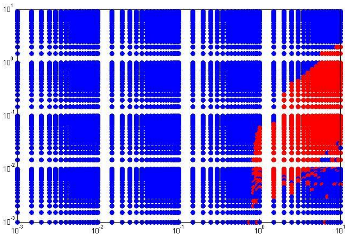
Figura 22 - Mapa de estabilidade Le=1,69 m (sem atrito)
