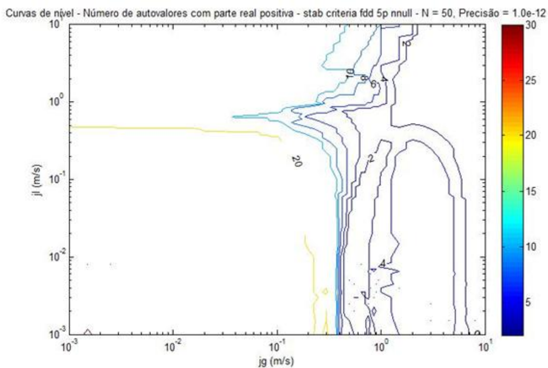
Figura 32 - Curva de nível Le=10 \text{ m} - Número de autovalores com parte real positiva
