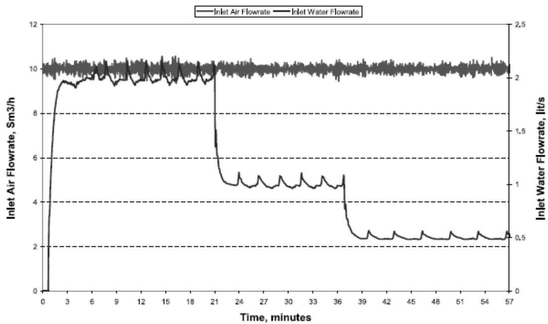
Figura 8 - Vazões de água e de ar utilizadas no experimento
