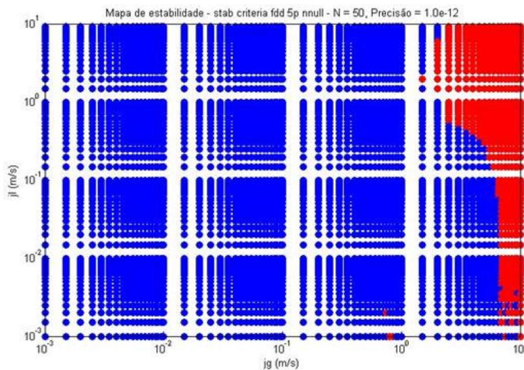
Figura 31 - Mapa de estabilidade Le=10 \text{ m}
